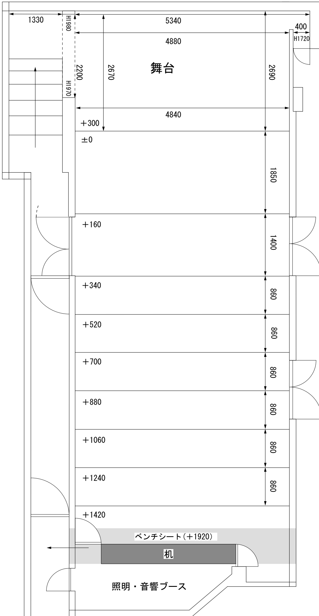
シアター711 平面図 1/50 (A4出力時)
